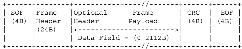
Fig. 13 FC Frame Format
